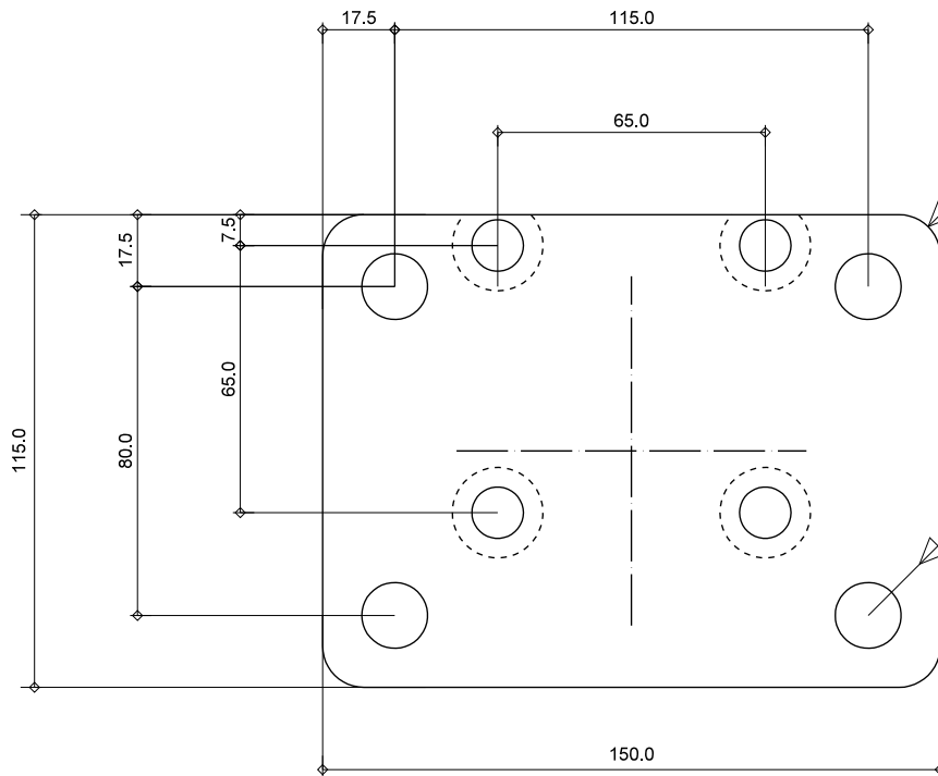
bovenaanzicht
